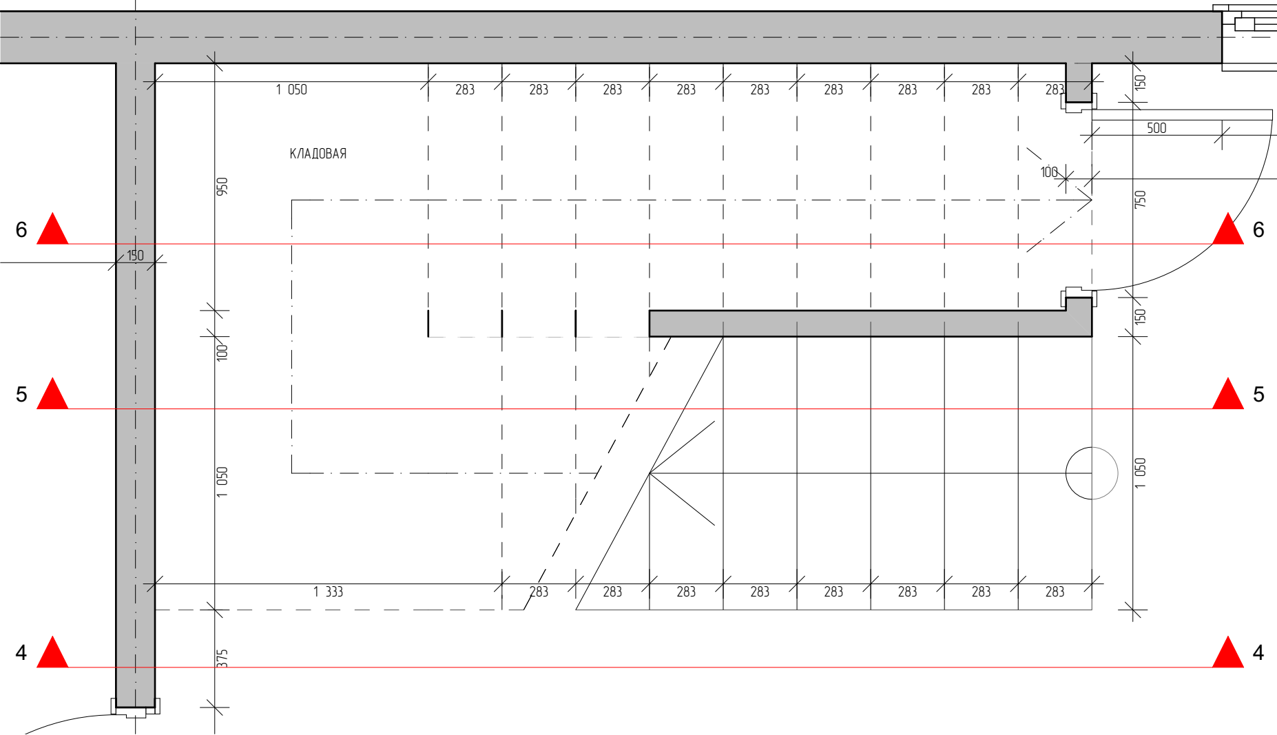
План лестницы М 1:20
