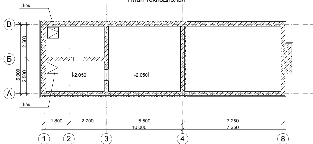
План техподполья
