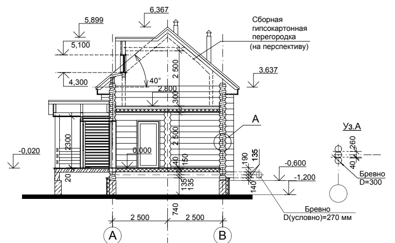
Разрез 1-1
